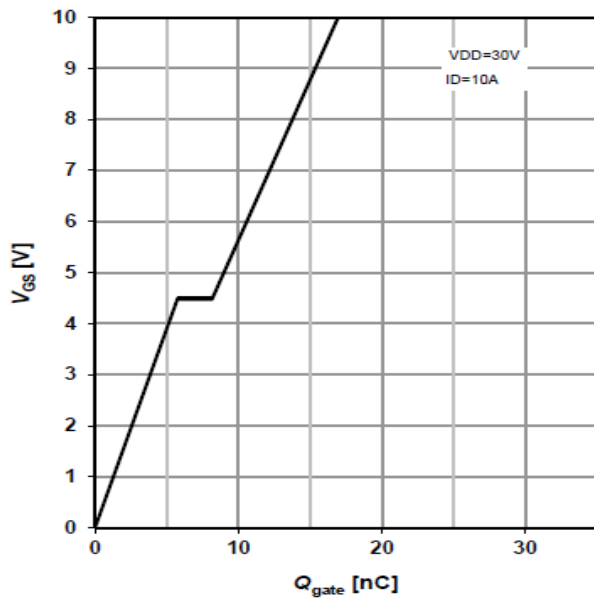
Typ.gate charge
